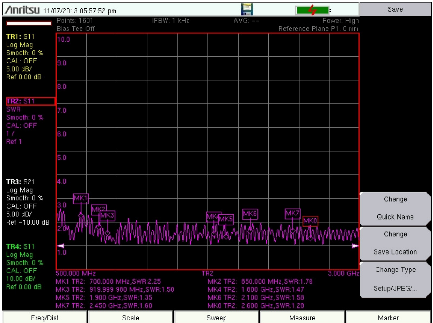
Figure 1 VSWR 500MHz – 3000MHz
